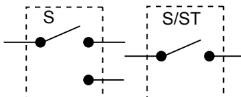
Позначення зовнішнього вимикача/перемикача на схемі
