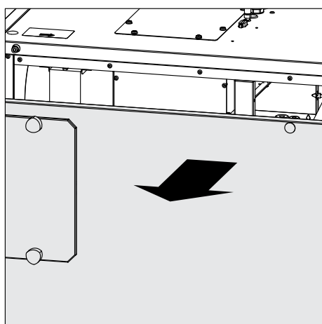
Підвісний стельовий монтаж
